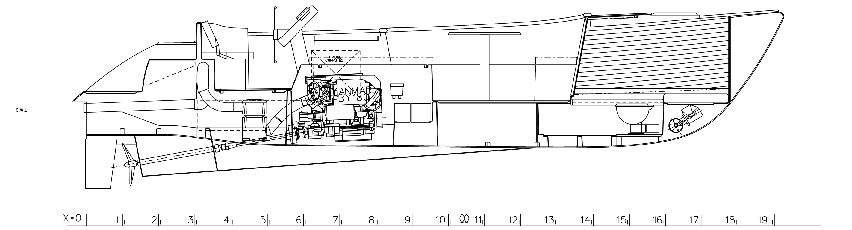
LONGITUDINAL SECTION
