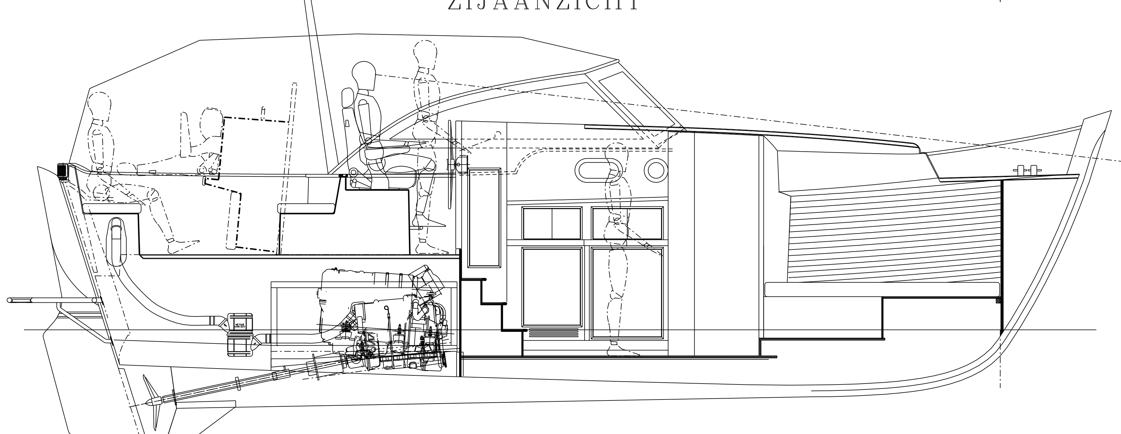
LANGSDOORSNEDE
