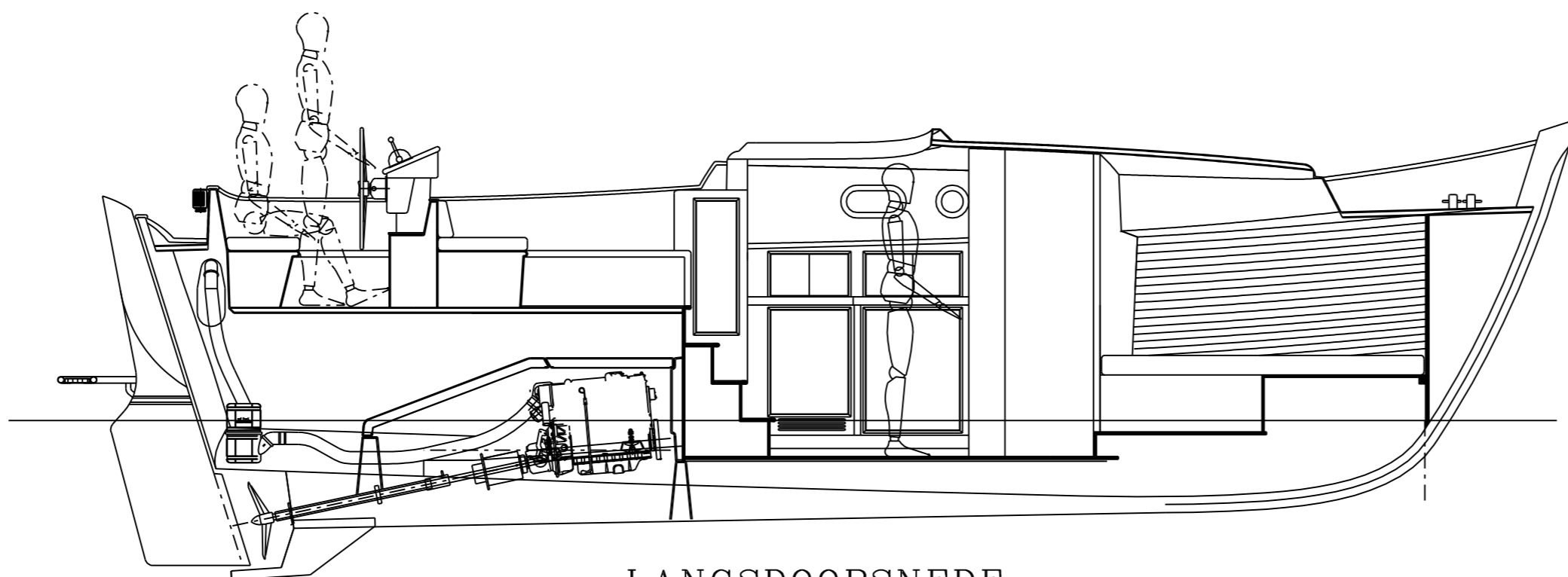
LANGSDOORSNEDE
