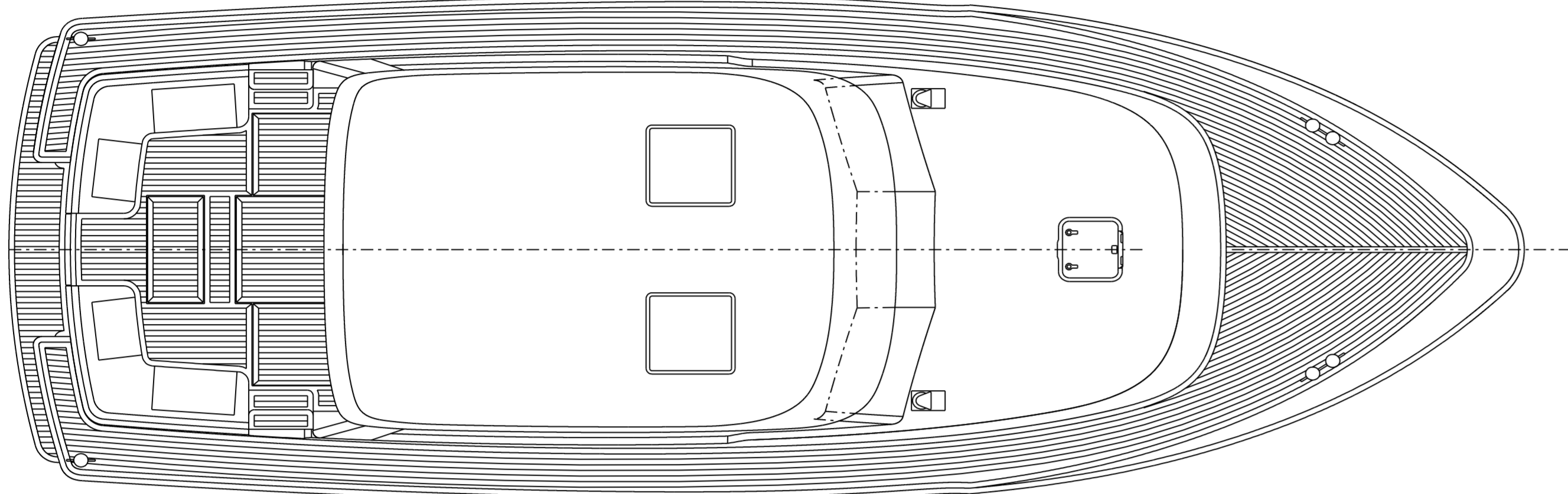
DEKAANZICHT
